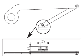
LEVA A COMPASSO R
