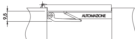
LEVA A COMPASSO R ET
