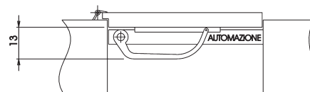
LEVA CURVA CON GUIDA AMBIDESTRA
